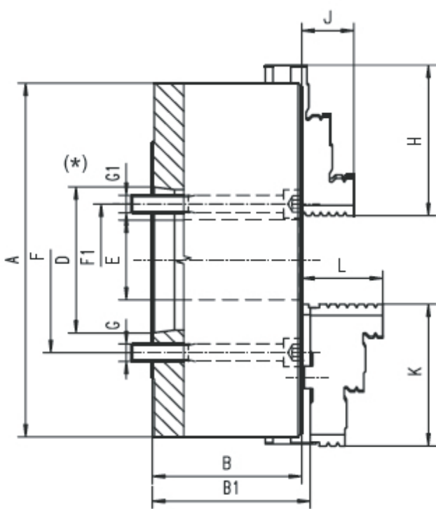
(*) Śruby wewnątrz stożka - typ A1
